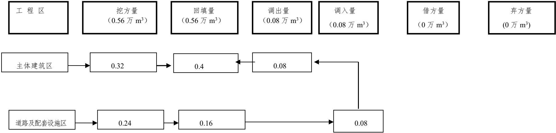
图 2-1 工程土石方平衡流程图
