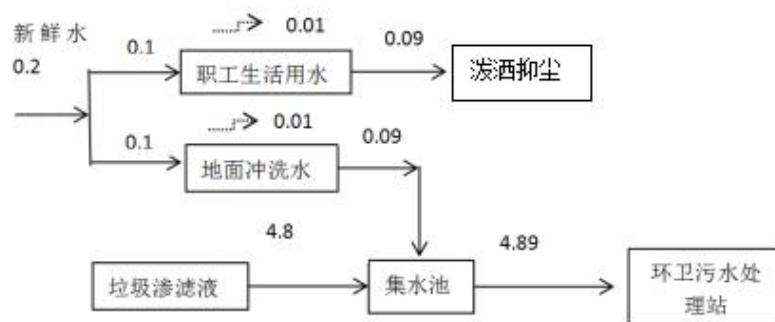
图 2 白水镇生活垃圾转运站水平衡图
