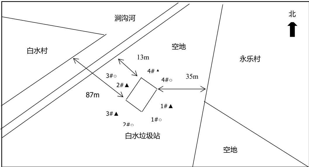
图 1 四邻关系图
